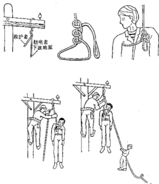
图 8 杆上或高处触电下放方法
